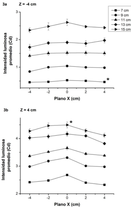
FIGURA 3. Perfiles de intensidad luminosa promedio en el plano X. 3a) Mínima (z = -4) y 3b) Máxima (z = 4). Los datos muestran el valor promedio ± error estándar. *Denota el perfil de intensidad luminosa promedio mínimo y máximo correspondiente.
